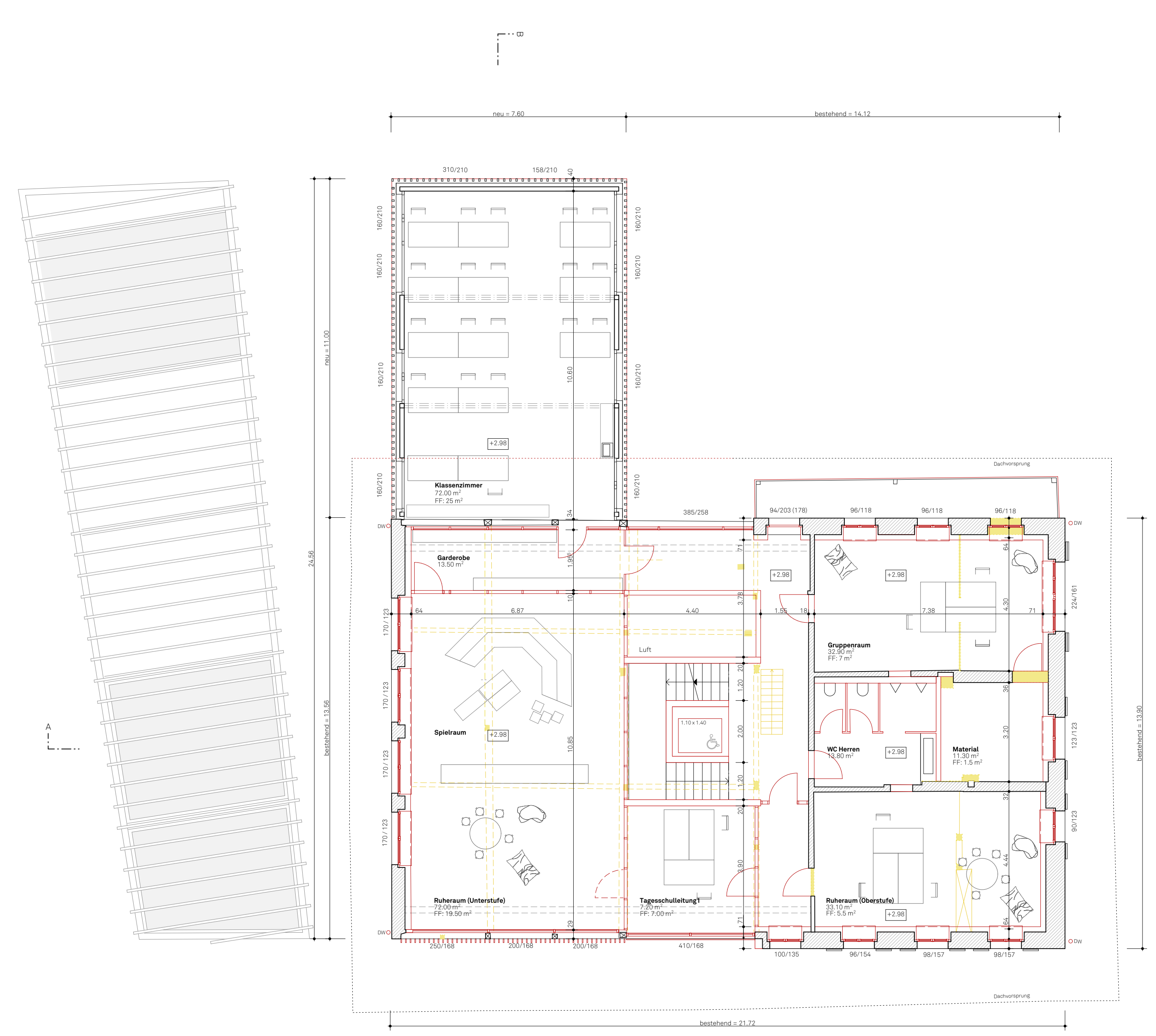
Obergeschoss
