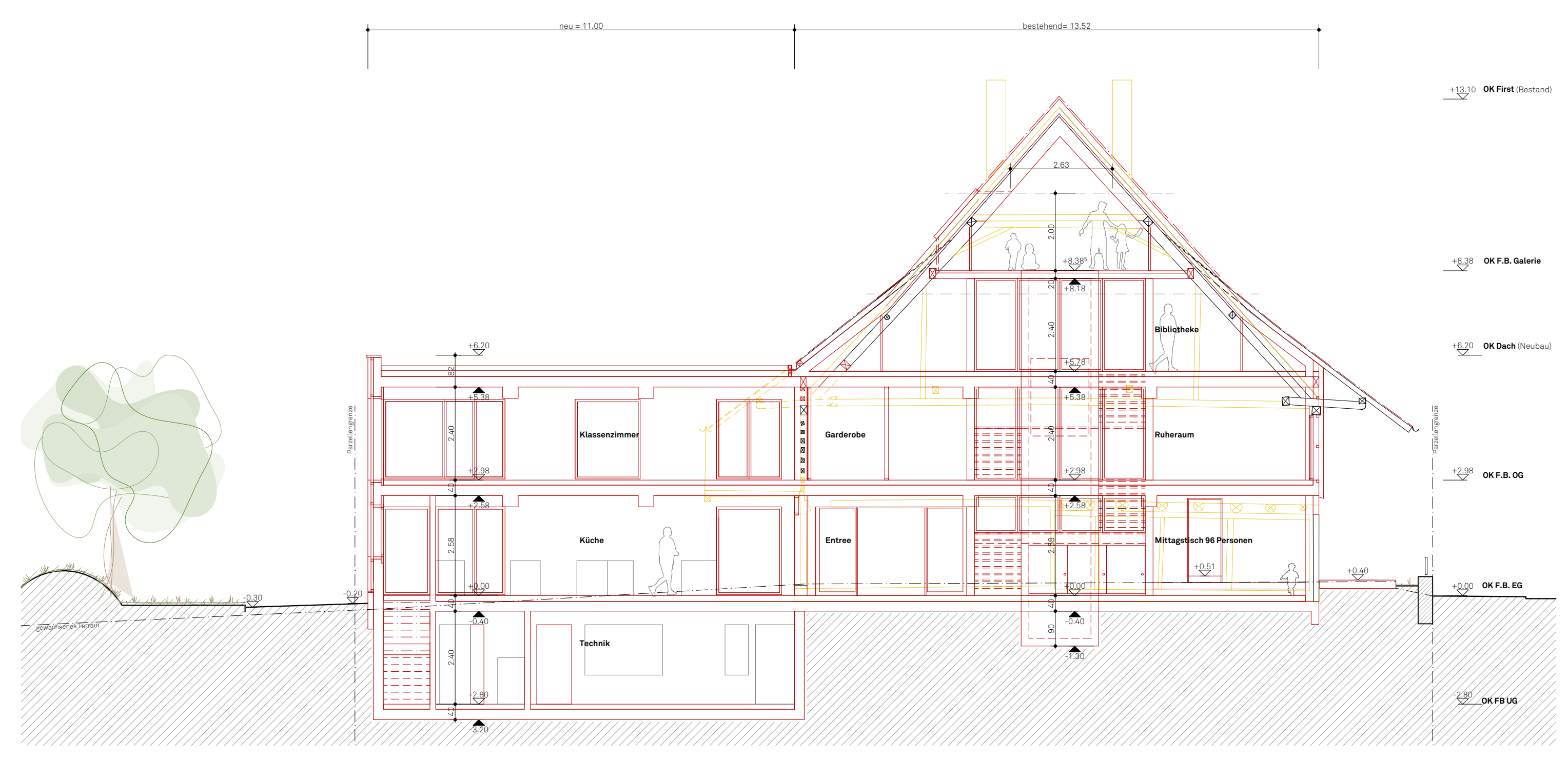
Schnitt B-B
