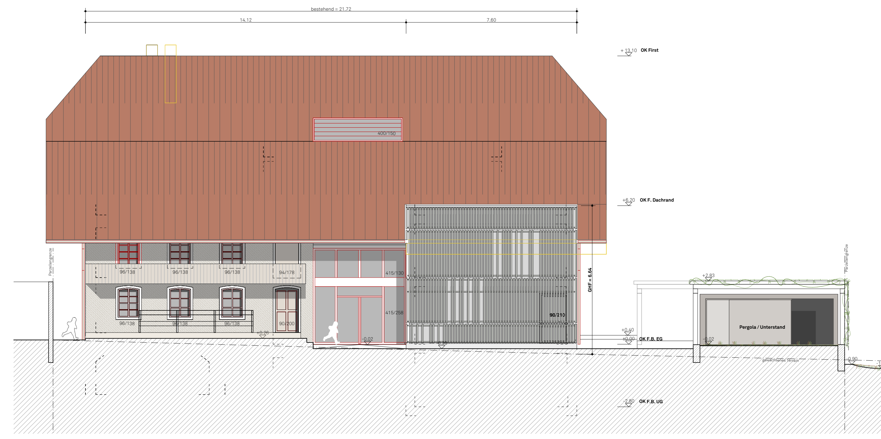
Fassade Nord
