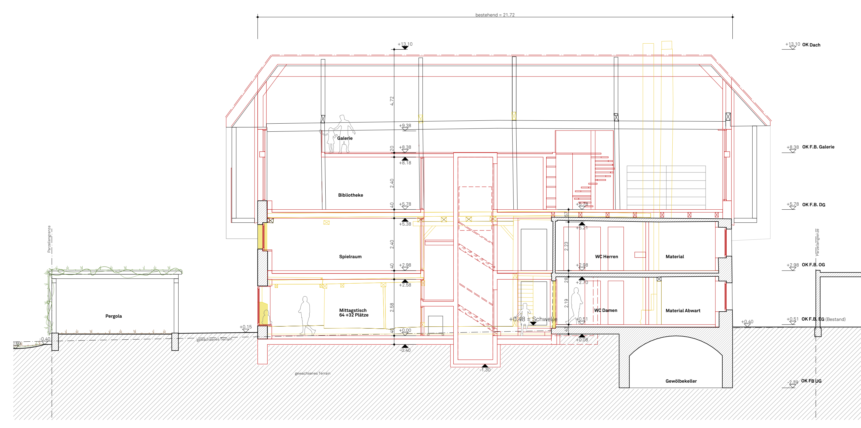
Schnitt A-A
